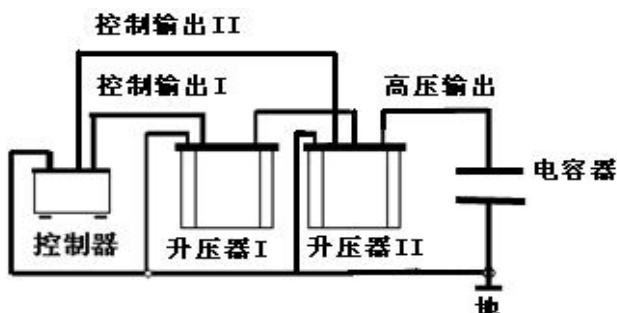
图 11 测量电容器的连线图
