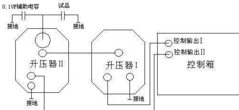
图4 (连线图)
